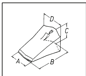
2) Type T
